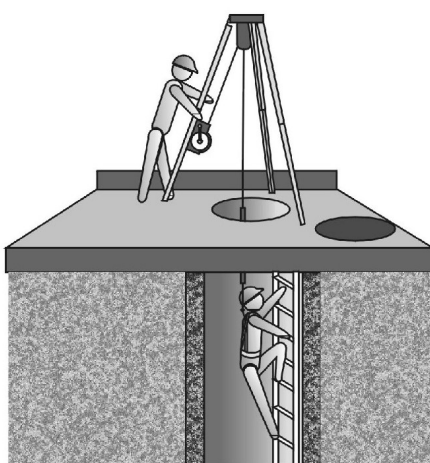
APLICACIÓN COMO SISTEMAS ANTICAÍDAS
