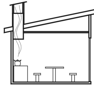
Sección transversal
